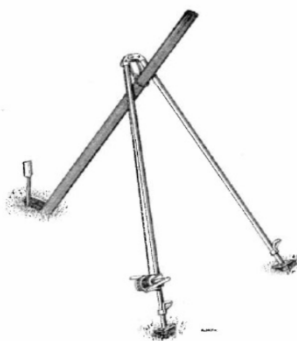
Figura 14 – Forma de içamento do cavalete articulado e guincho manual
