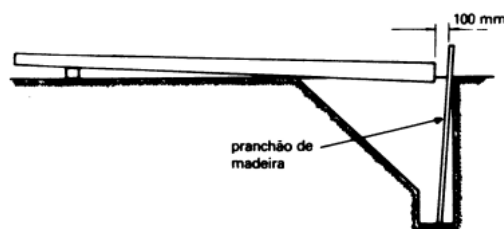
Figura 11 - Posição da tábua no lado oposto do cachimbo
