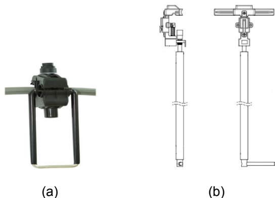
Figura 2 – a) Conector perfurante com estribo revestido; b) Bastão com cabeçote para aplicação do conector perfurante com estribo à distância
