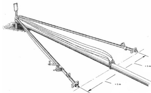
Figura 13 – Afastamento do cavalete em relação ao eixo do poste
